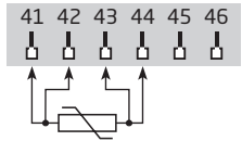
WTH & Lin R, 4-Leiter
